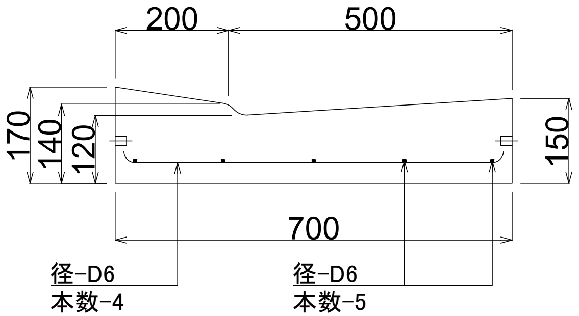
断面図
