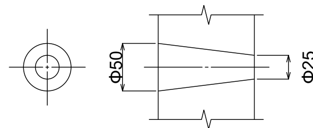
排水孔詳細図
