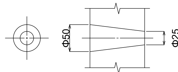
排水孔詳細図
