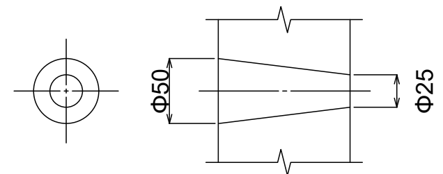
排水孔詳細図
