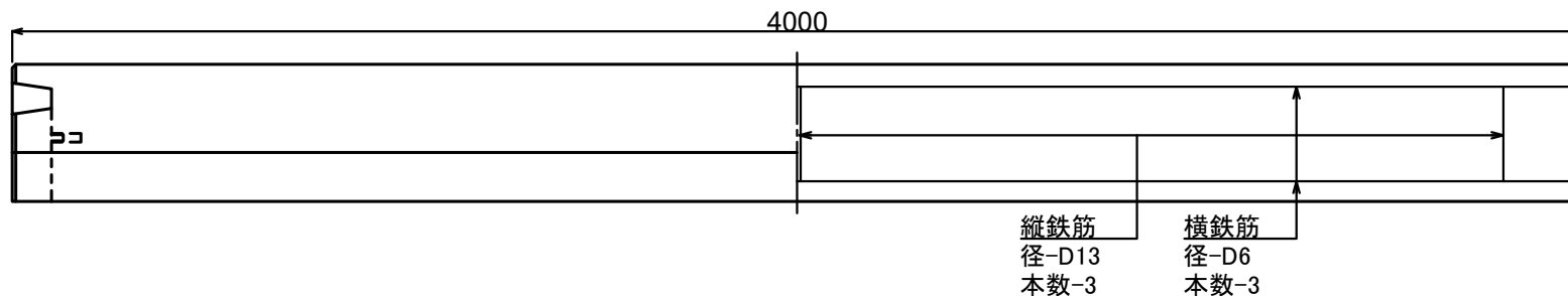
平面図
