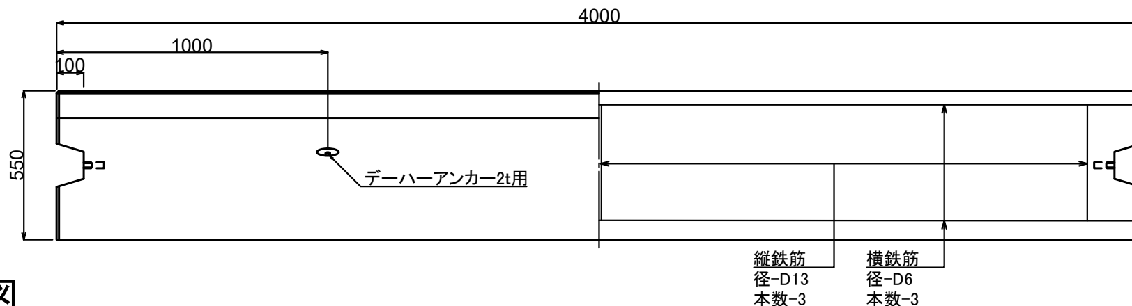
平面図
