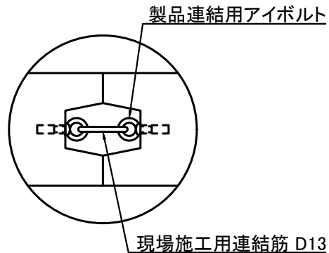
連結部詳細図
