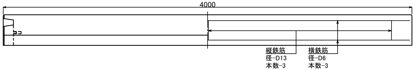
平面図
