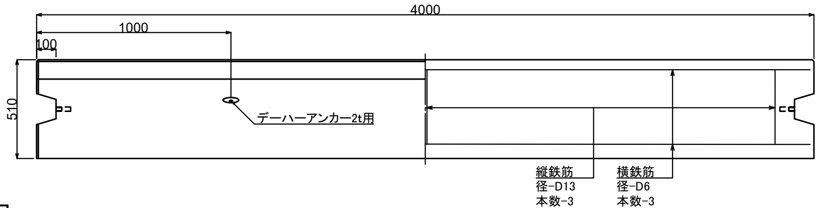
平面図
