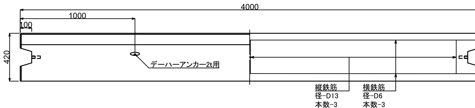
平面図
