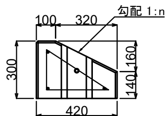
側面図
