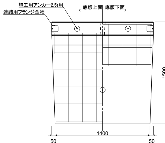
上面図
